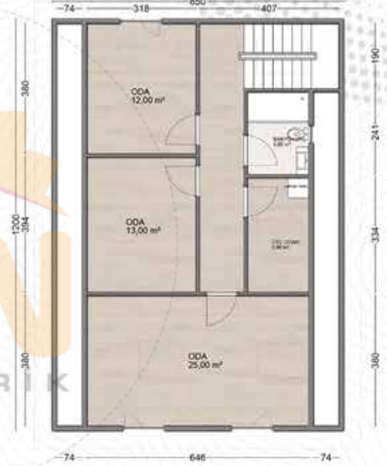
BİRİNCİ KAT PLANI
