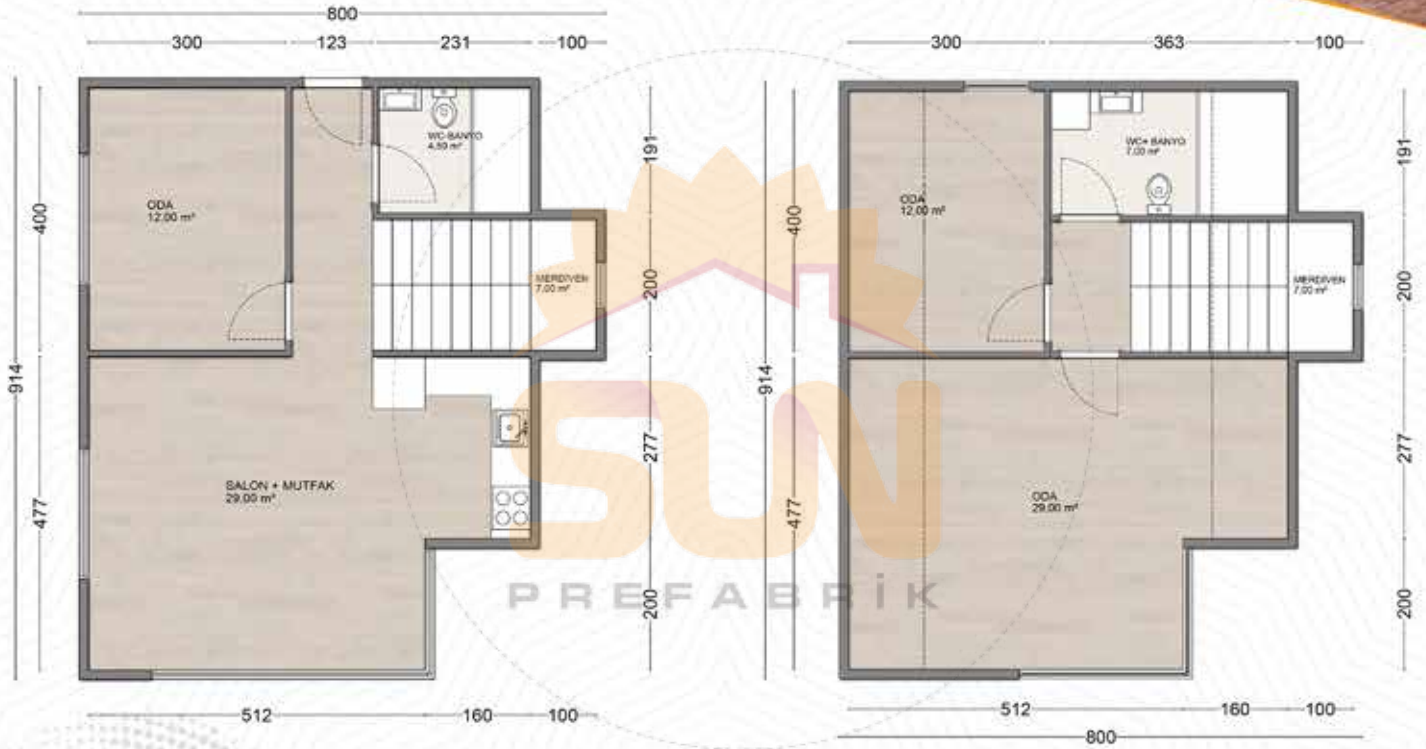
ZEMİN KAT PLANI
